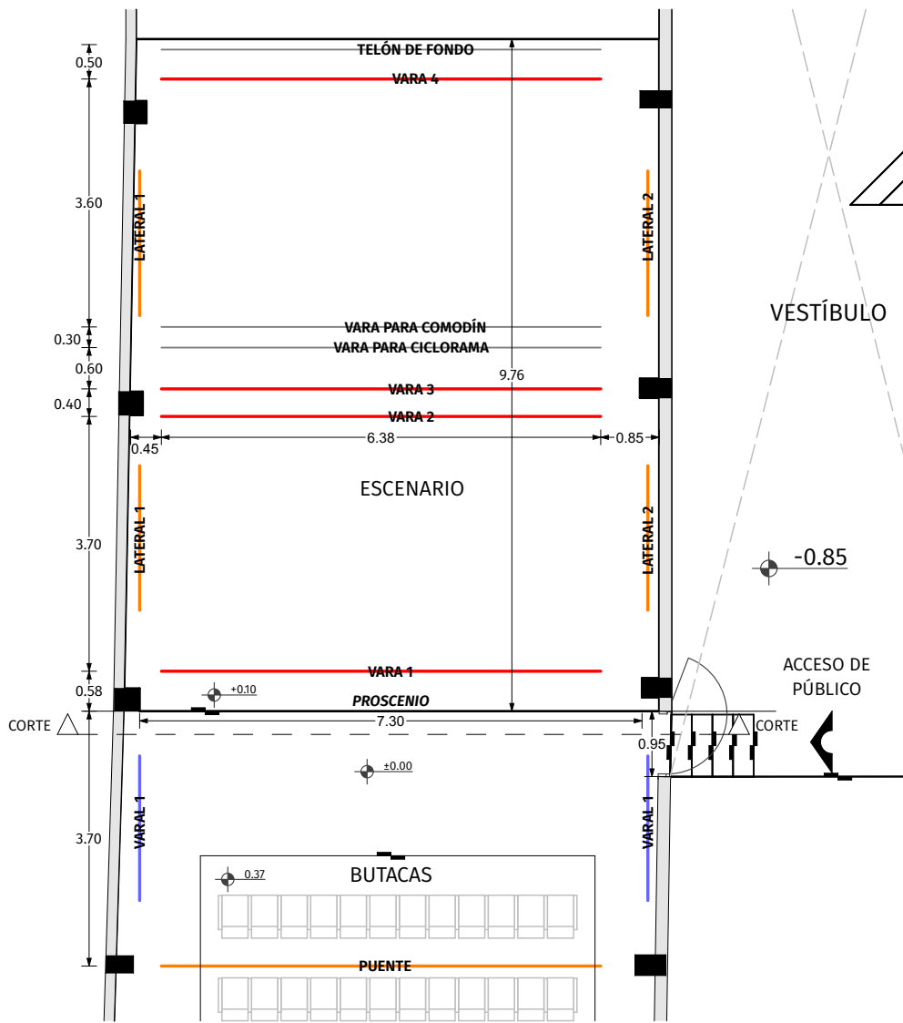
0. Planta de iluminación 1:100
